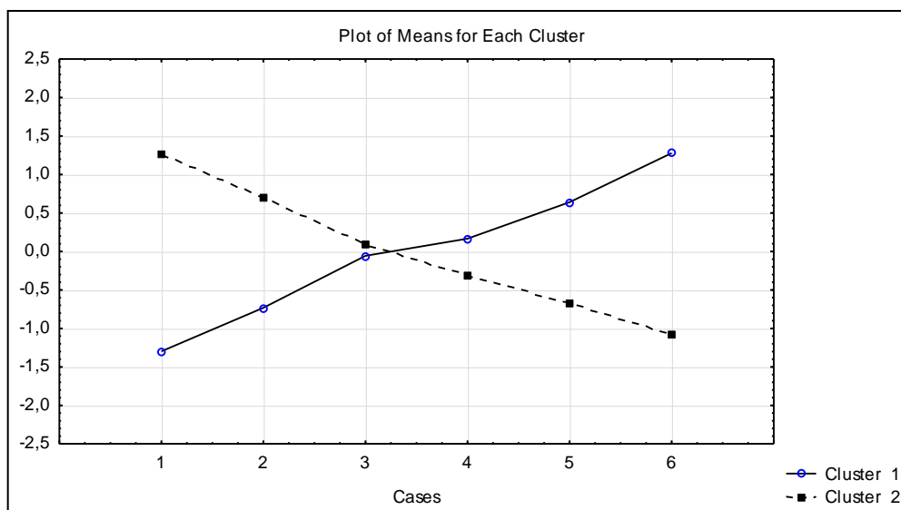
Рис. 6. Кластеризація статей витрат домогосподарств Польщі за 2013-2018 рр. методом k-середніх (Авторська розробка)
