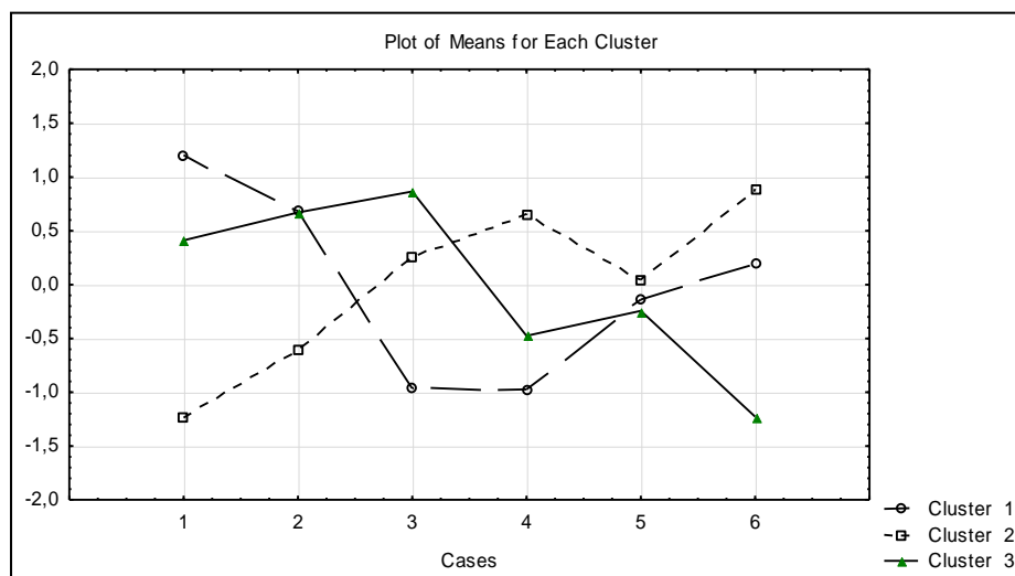
Рис. 5. Кластеризація статей витрат домогосподарств України за 2013-2018 рр. методом k-середніх (Авторська розробка)
