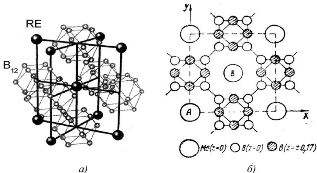
Рис.1. Кристаллическая структура додекаборидов редкоземельных металлов типа UB_{12} в пространстве a) и в проекции на плоскость XOY б)
